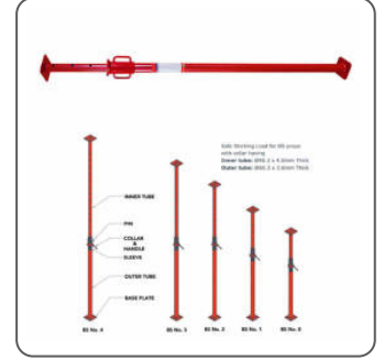
دعامات حديد Iron Props
